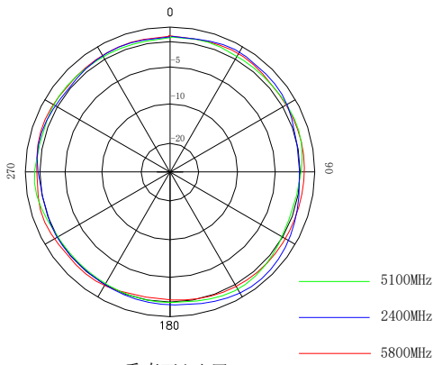
垂直面方向图 Vertical Pattern
