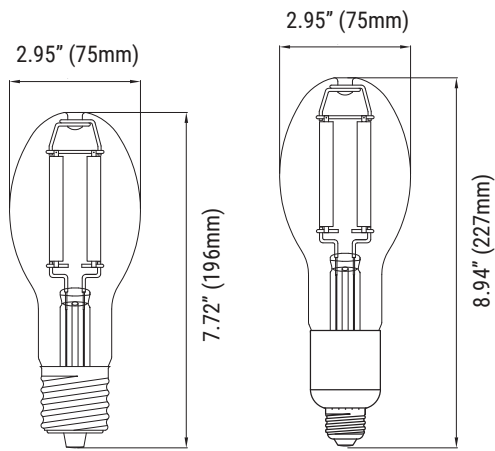
E23.5 Lamp 20 Watt: 0.37-lbs
