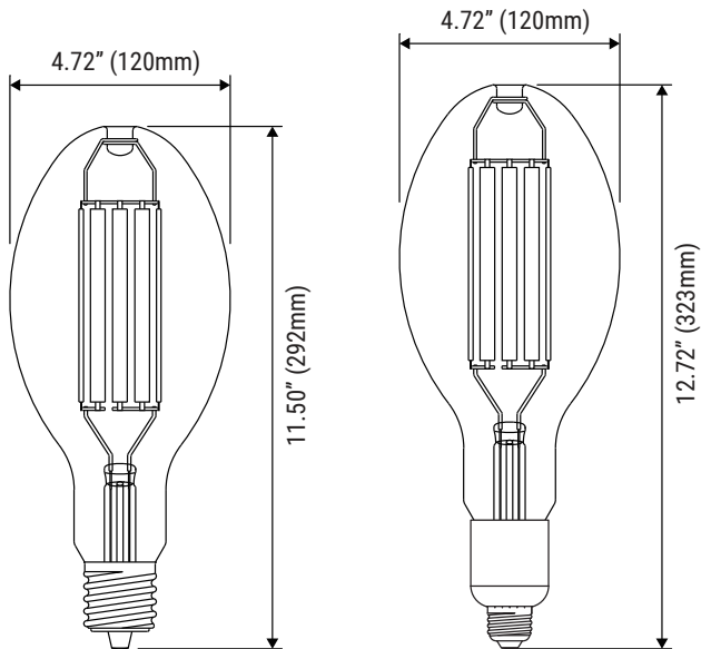
E37 Lamp 55 Watt: 0.62-lbs
