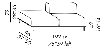
elemento penisola / peninsula unit 195
