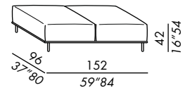
elemento isola / island unit 155
