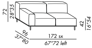
terminale / end unit 175
