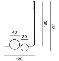
SUPERB-ALL HORIZONTAL L 120 Ø60-Ø20
