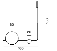
SUPERB-ALL HORIZONTAL L 160 Ø60-Ø30
