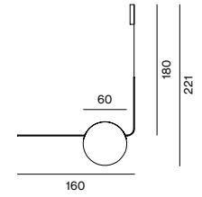
SUPERB-ALL HORIZONTAL L 160 Ø60
