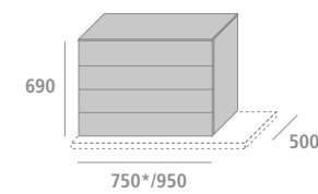
Cassettiera per basamento e su ruote in melaminico con quattro cassetti Drawer unit on base and on wheels in melamine with four drawers
