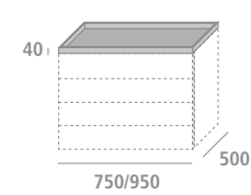
Top opzionale in melaminico larice carbone con fondo rivestito in cuoio rigenerato, per cassetteria su basamento o su ruote Optional top in coal larch melamine with bottom part covered with regenerated leather, for drawer units on base or on wheels
