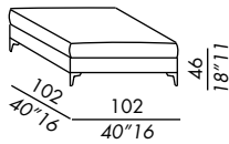
pouf
