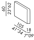
bracciolo / armrest SLIM 60
