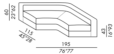
elemento elbow / elbow unit 195
