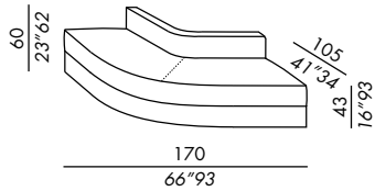
elemento elbow aperto / open elbow unit 170
