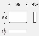
Bracciolo / Armrest / 15
