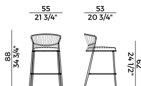
923/S sgabello \ barstool
