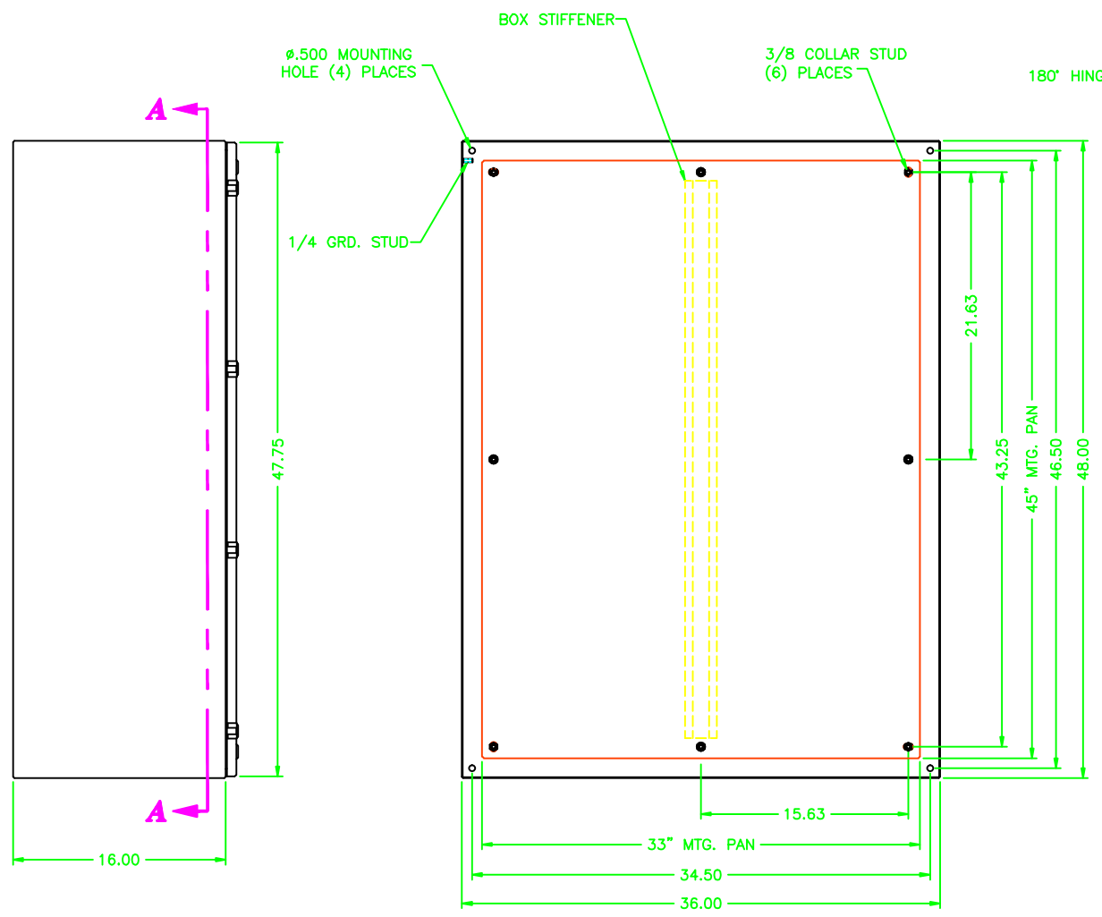
SECTION A-A
