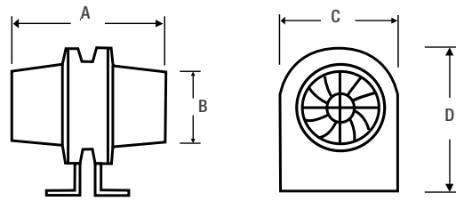
Dimensions - SF150
