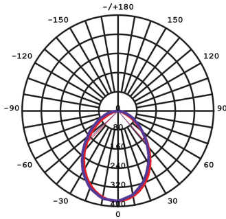
S9041 TC 3000K
