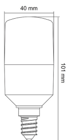
LT407 E14
