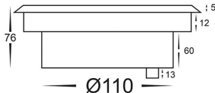
Cutout without Canister Ø136 Ø160
