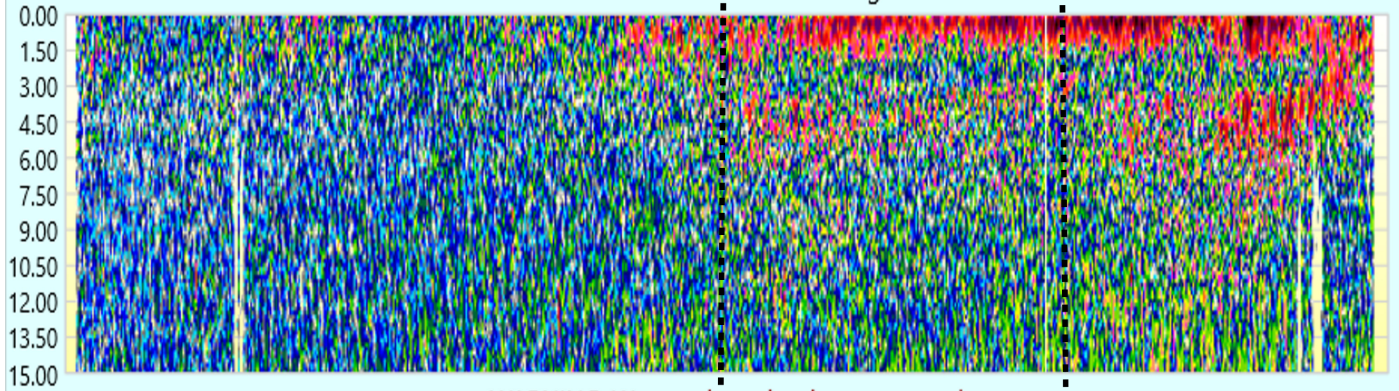
SNDG00027 - Sub Bottom Echogram
