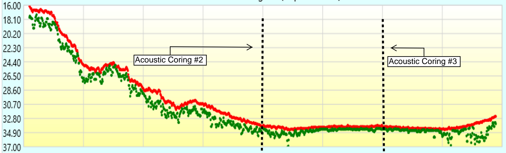
SNDG00027 - Echogram (Depth vs Time)
