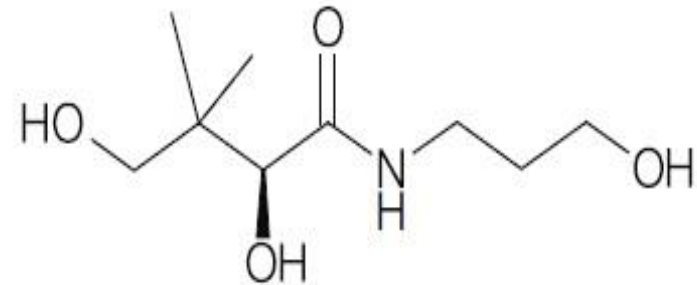
D-Panthenol
