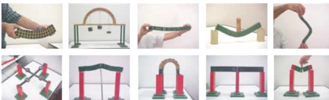
Figura 2.18 – Yopanan Rebello: modelos estruturais qualitativos
