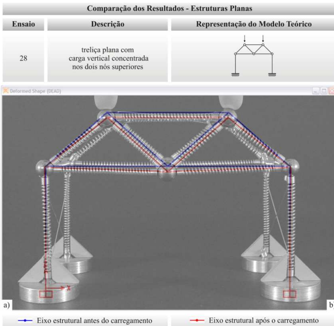
Figura 5.28 – Sobreposição das imagens: estruturas planas - ensaio 28 a) Imagem do modelo deformado, b) Deformada gerada pelo software impressa em transparência
