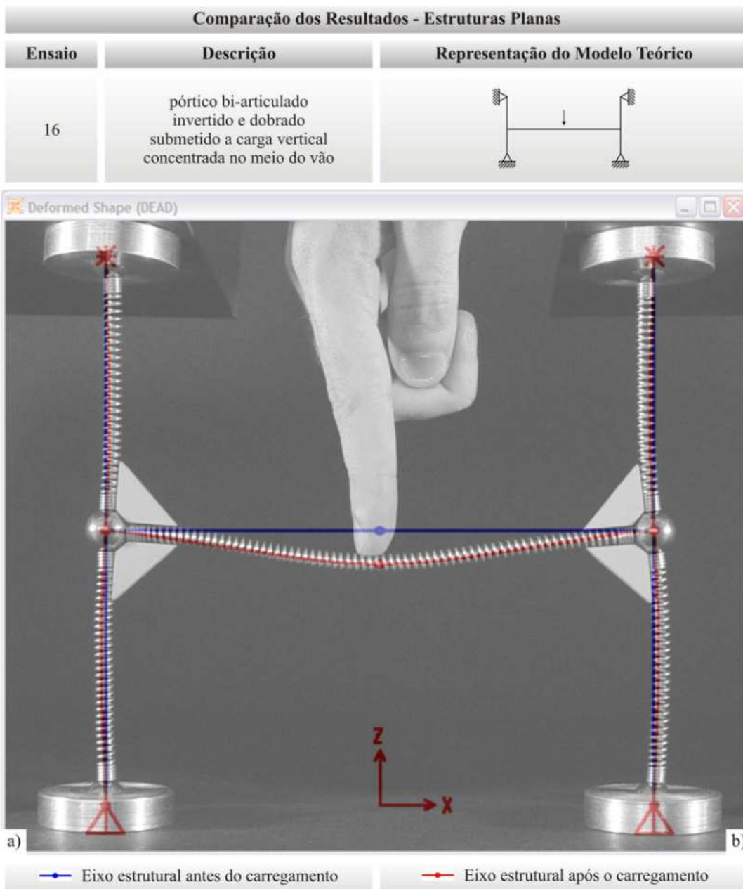
Figura 5.16 – Sobreposição das imagens: estruturas planas - ensaio 16 a) Imagem do modelo deformado, b) Deformada gerada pelo software impressa em transparência
