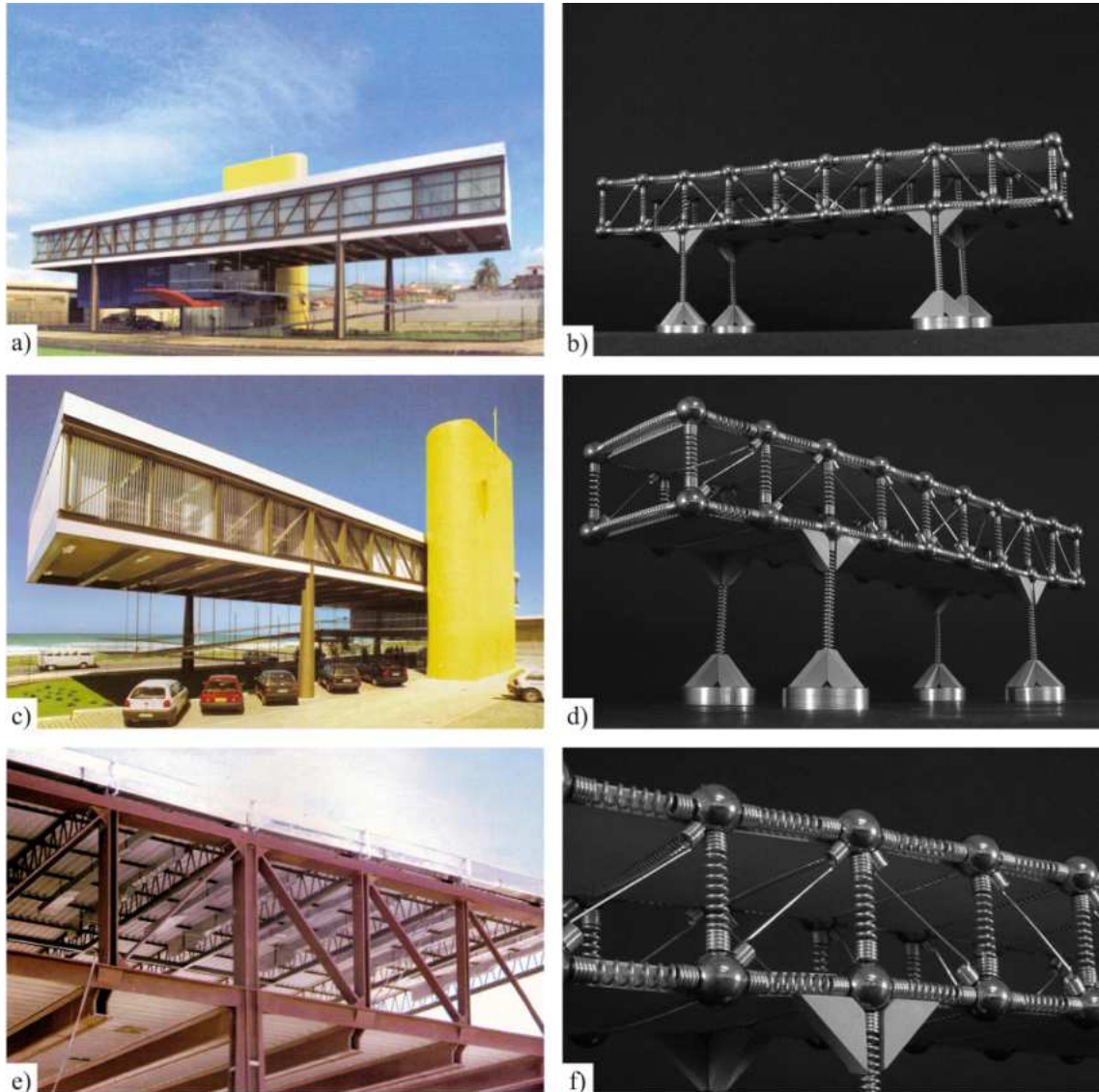
Figura 7.3 –Tribunal de Contas de Alagoas representado com a Maquete Estrutural Fonte: a), c), e) DIAS, 2001.
