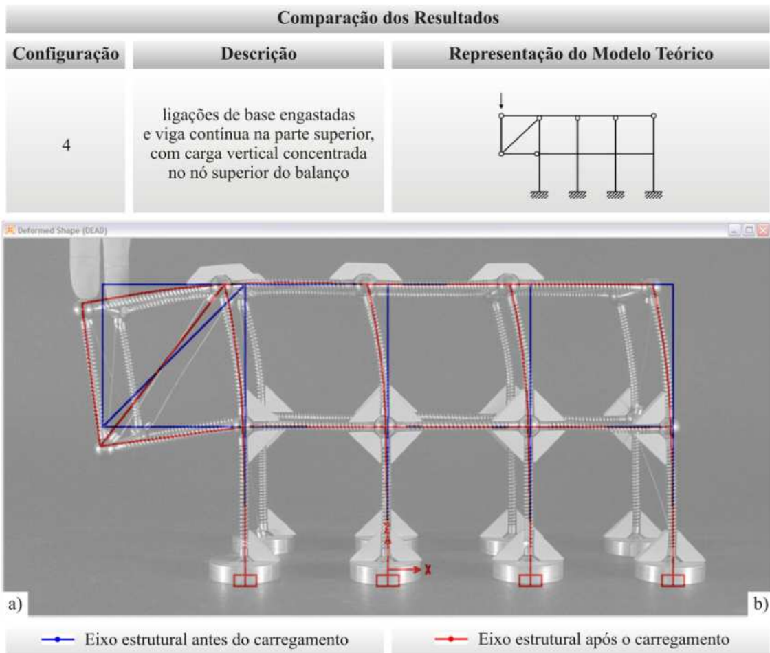
Figura 6.8 – Sobreposição das imagens: configuração 4 a) Imagem do modelo deformado, b) Deformada gerada pelo software impressa em transparência
