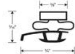
GSK223
