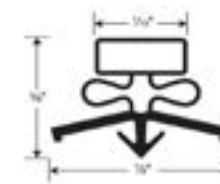
GSK139
