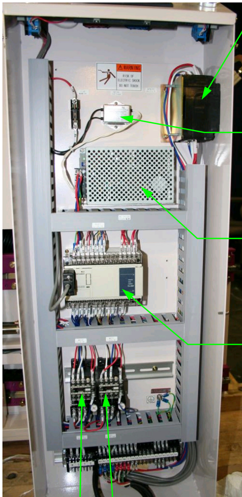
Contact Blower CPS30-402
