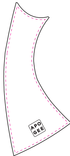
latérale droite/ right side panel
