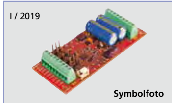
I / 2019 36125 PIKO SmartDecoder 4.1 für G-Lokomotiven PIKO SmartDecoder 4.1 Kit for G scale locomotives
