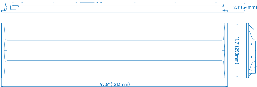
TDHE 14 LS42 - 1' x 4' Troffer
