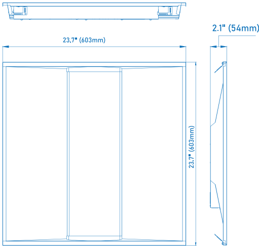
TDHE 22 LS42 - 2' x 2' Troffer
