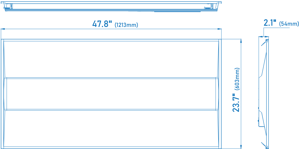
TDHE 24 LS51 - 2' x 4' Troffer
