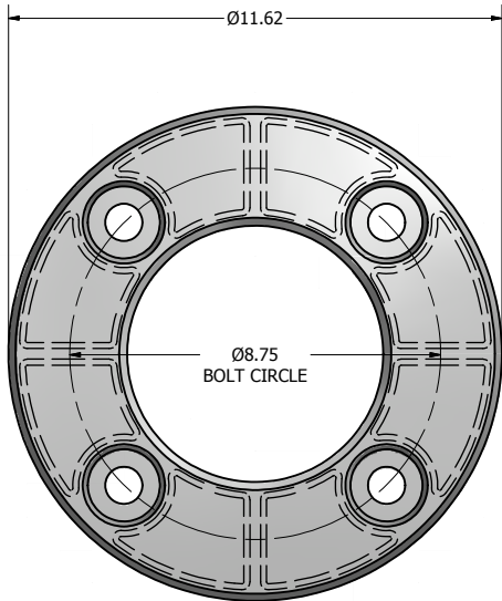
Ø11.62 X 1.88 THK. BASE CASTING
