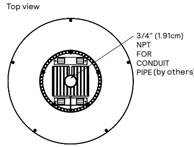
Direct Pendant mount
