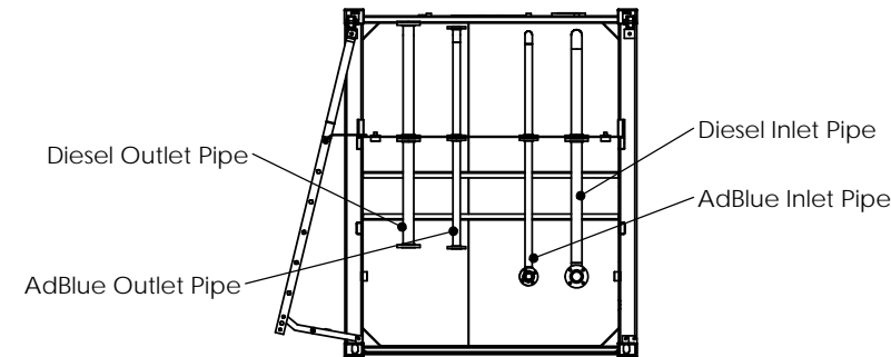
剖面 D-D
