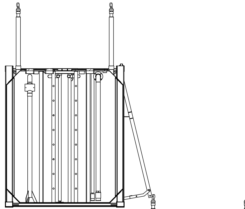
剖面 D-D
