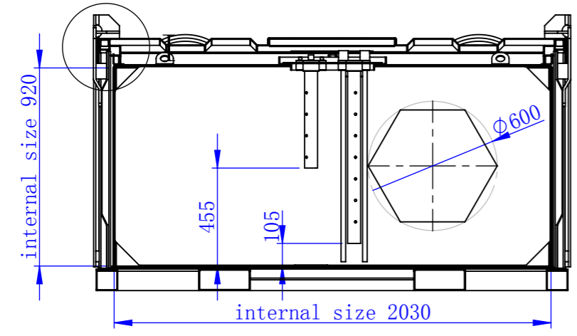
B-B
