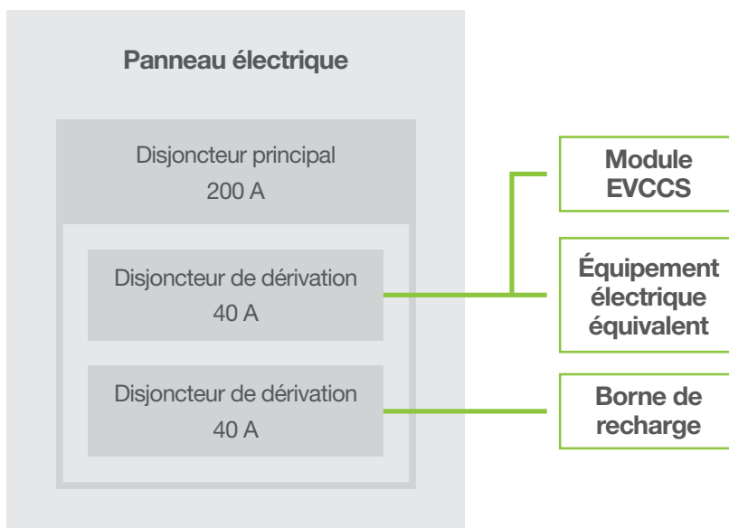
Figure 5 : Exemple d'une mesure de courant de type « Parallèle »
