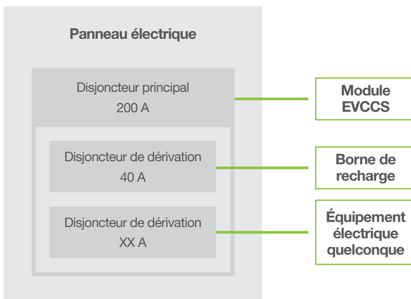
Figure 4 : Exemple d'une mesure de courant de type « Amont »
