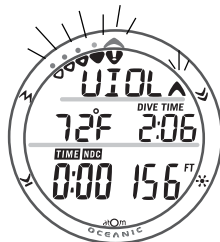
Fig. 142 - FREE DIVE MAIN (During DECO)
