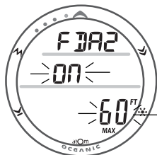
Fig. 133 - SET FREE DEPTH ALARM 2
