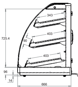
End Elevation
