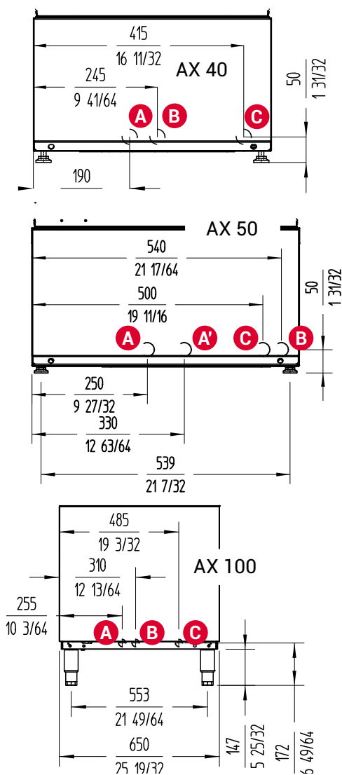
Abb. 1: Maschinenanschlusspunkte
