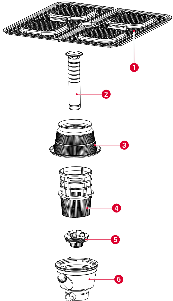
Abb. 3: Maschinenfilter
