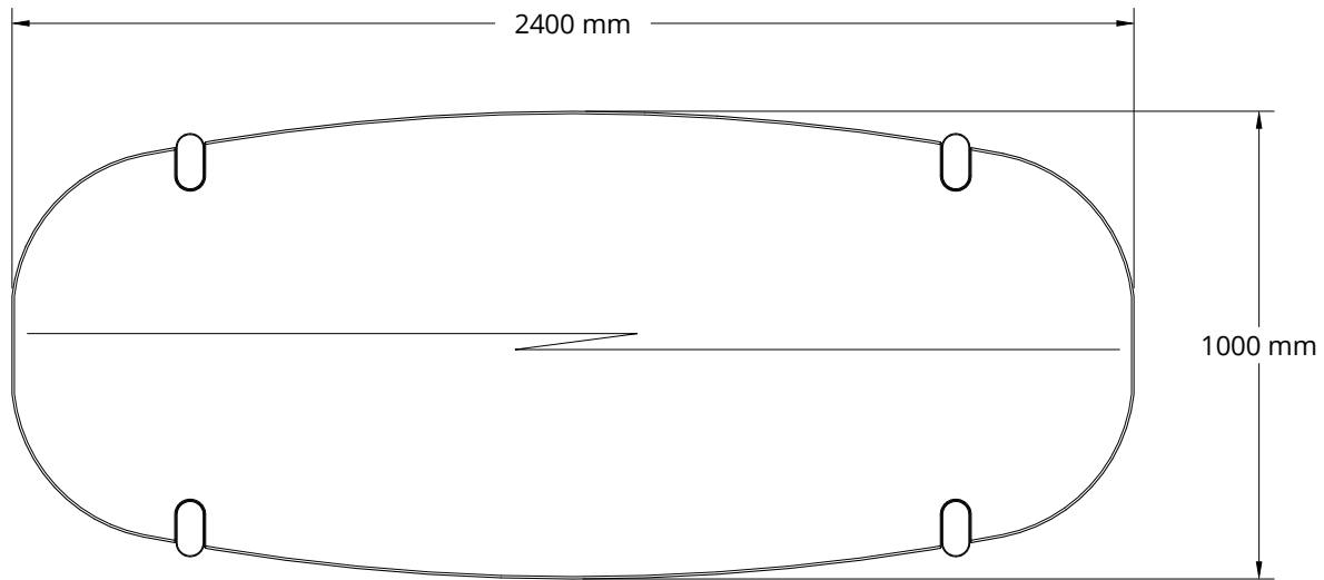
TAMPAK DEPAN
