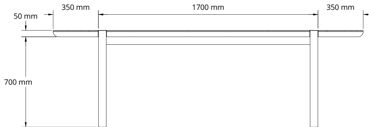
TAMPAK DEPAN
