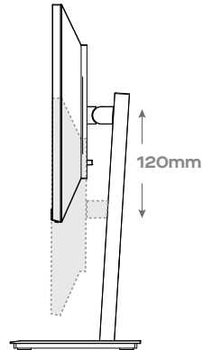
Plage de hauteur 120mm ( \pm 5.0 mm)
