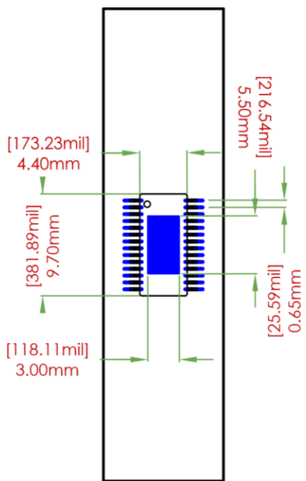
FOOTPRINT DIMENSIONS
