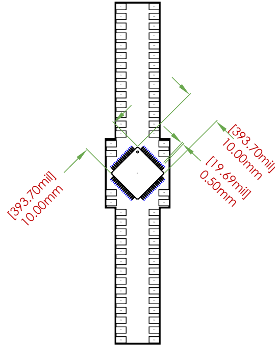
FOOTPRINT DIMENSIONS
