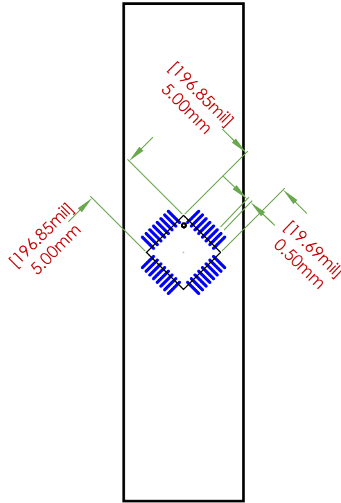
FOOTPRINT DIMENSIONS
