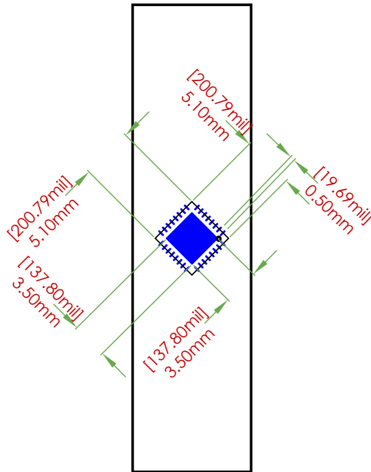
FOOTPRINT DIMENSIONS
