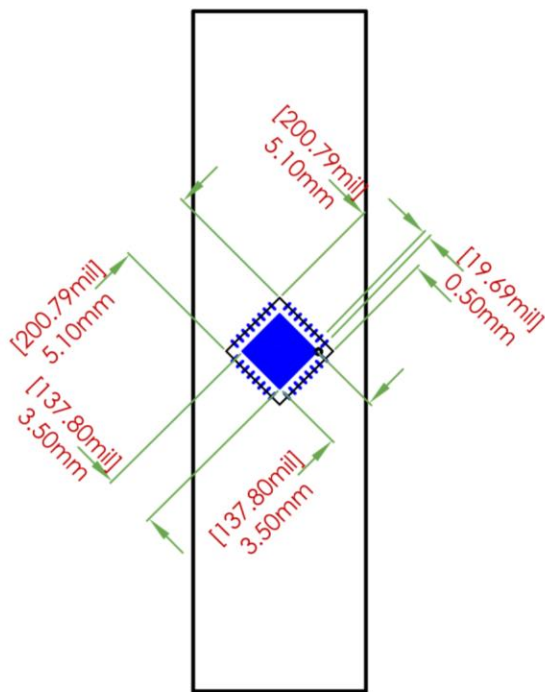
FOOTPRINT DIMENSIONS
