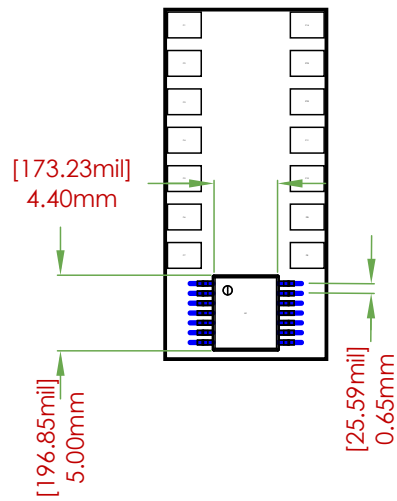
FOOTPRINT DIMENSIONS
