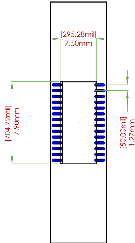
FOOTPRINT DIMENSIONS
