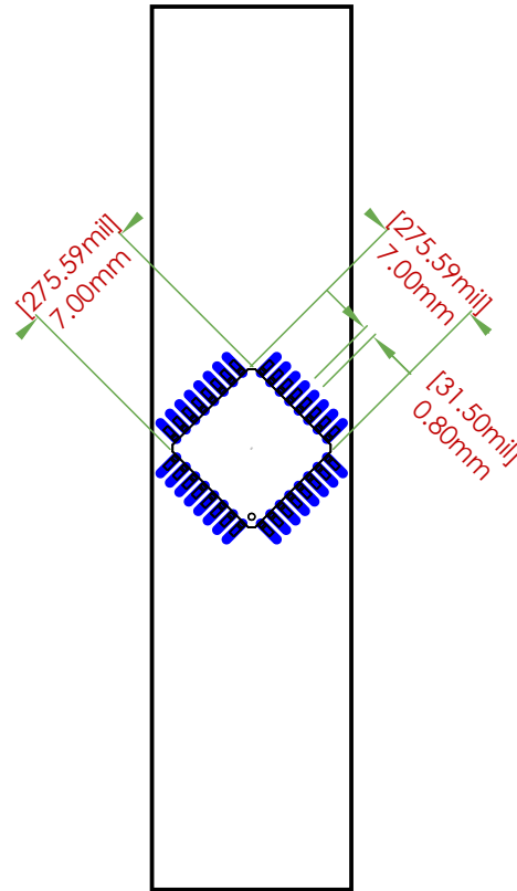
FOOTPRINT DIMENSIONS
