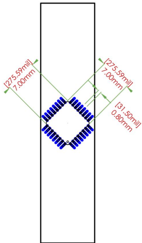
FOOTPRINT DIMENSIONS
