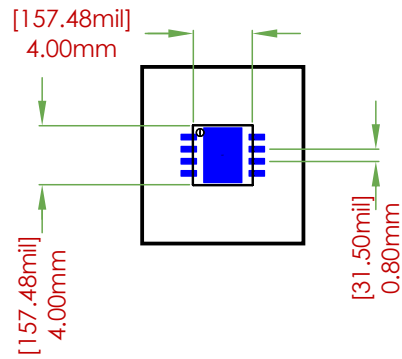
FOOTPRINT DIMENSIONS
