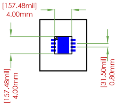
FOOTPRINT DIMENSIONS
