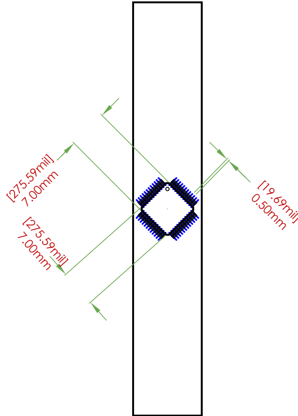
FOOTPRINT DIMENSIONS
