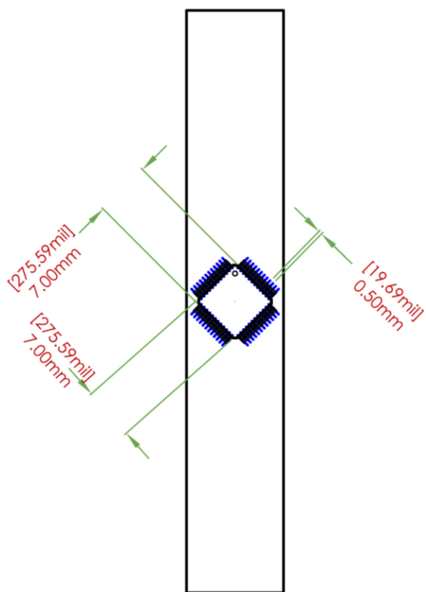
FOOTPRINT DIMENSIONS
