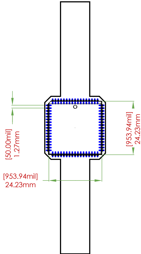
FOOTPRINT DIMENSIONS
