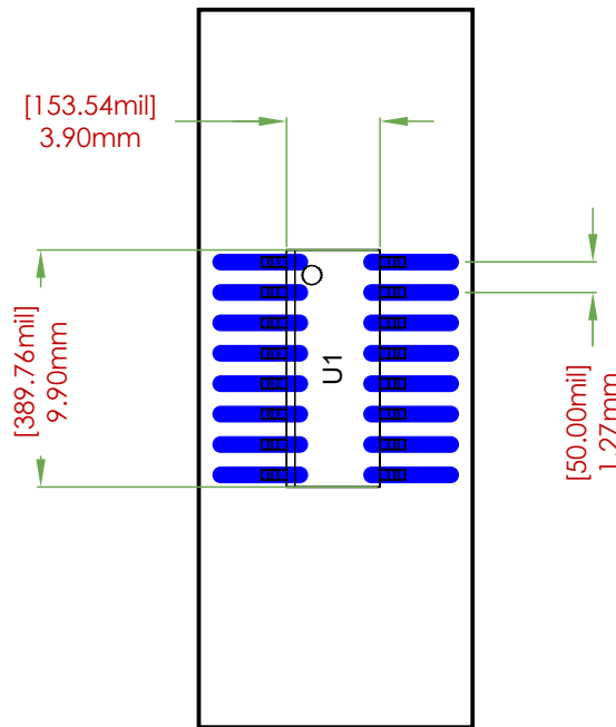
FOOTPRINT DIMENSIONS
