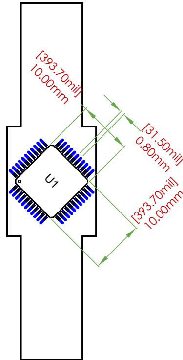
FOOTPRINT DIMENSIONS
