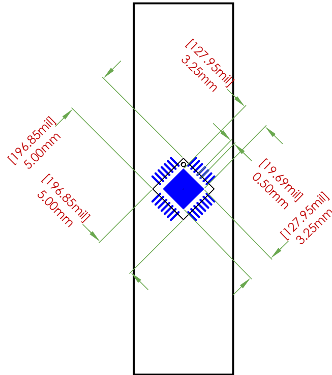
FOOTPRINT DIMENSIONS
